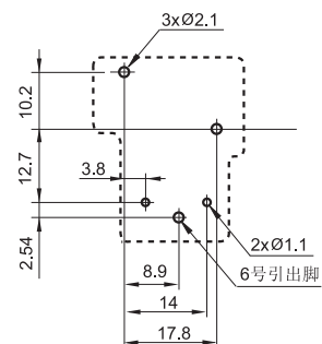
安装孔尺寸
