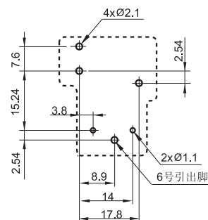
安装孔尺寸
