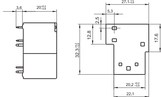
外形图
